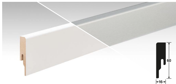
Akzent-Sockelleiste ASL 60 (weiß, dekoridentisch, edelstahl, anthrazit) 16 x 60 x 2380 mm
