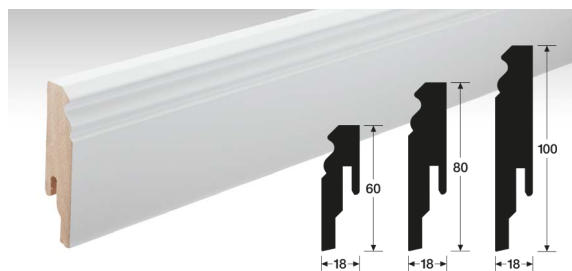
Hamburger Sockelleiste HSL 60 | 80 | 100 (weiß) 18 x 60 x 2380 mm 18 x 80 x 2380 mm 18 x 100 x 2380 mm
